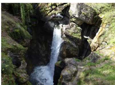
Le caldaie del torrente Devero
